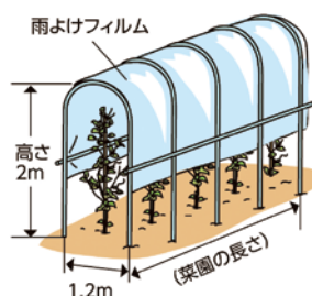
図3 雨よけ
